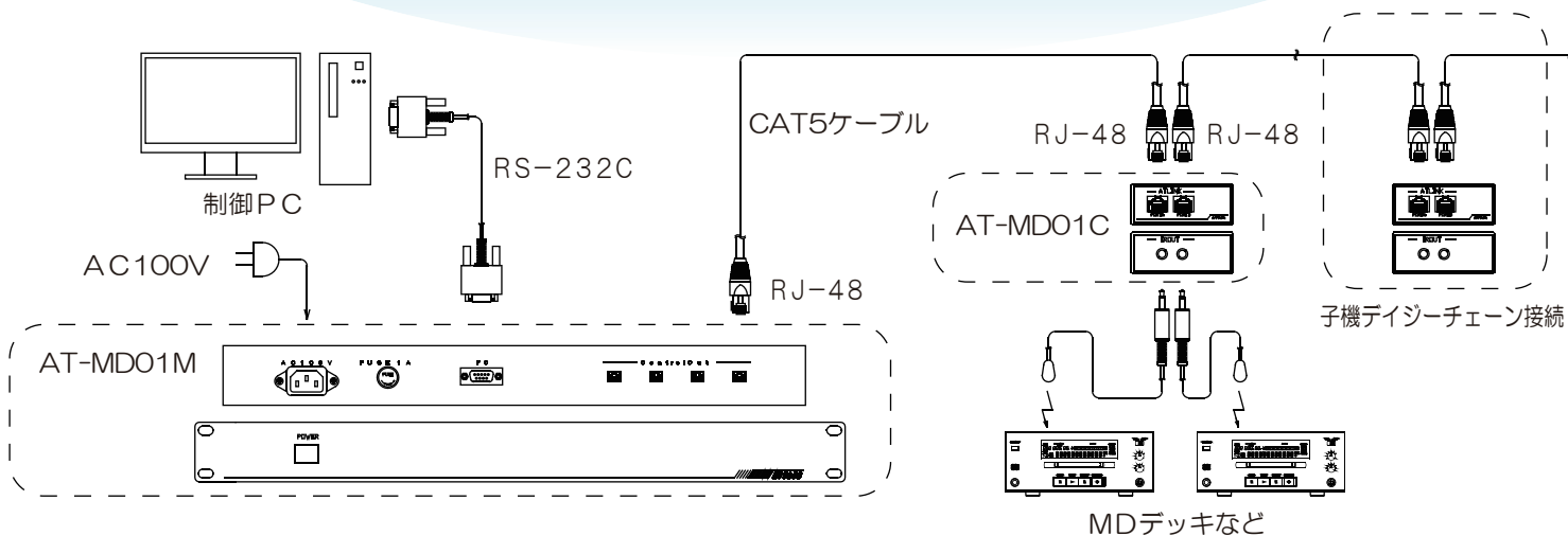
子機1台につきIRケーブル2本付属
